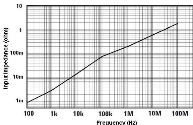
图 3.b CP8030H 输入阻抗 VS 频率曲线
