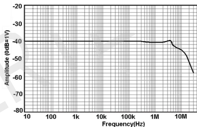
图 13 CP8500A 幅频曲线
