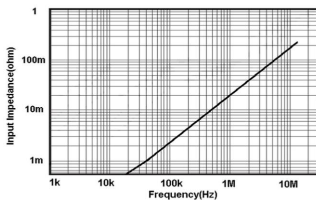
图 9 CP8150A 输入阻抗 VS 频率曲线
