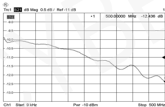
图 1 频响曲线
