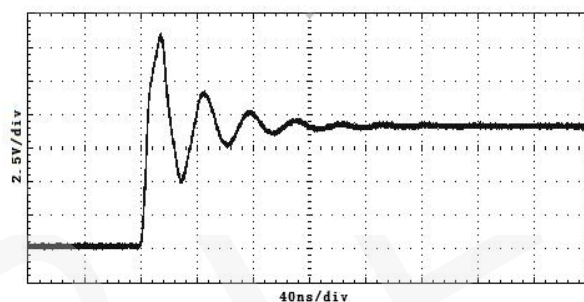
添加输入延长线(CK-301)的波形
