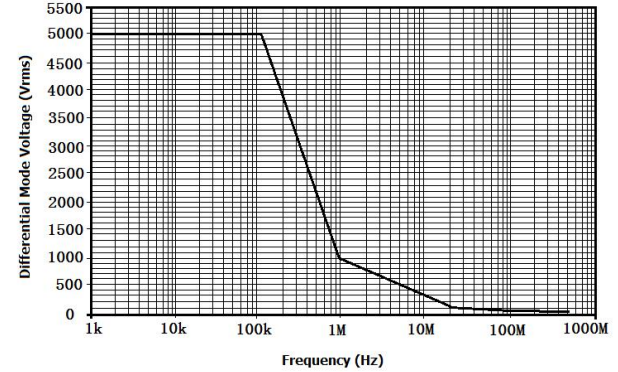
图 4 DP6700B 最大差模电压 VS 频率
