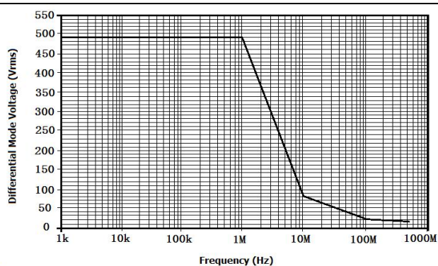
图 1 DPX6070B 最大差模电压 VS 频率
