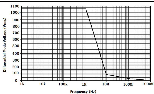
8 图 2 DPX6150B 最大差模电压 VS 频率
