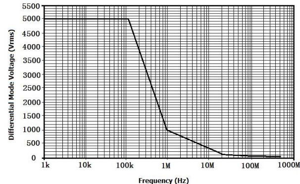
图 4 DPX6700B 最大差模电压 VS 频率
