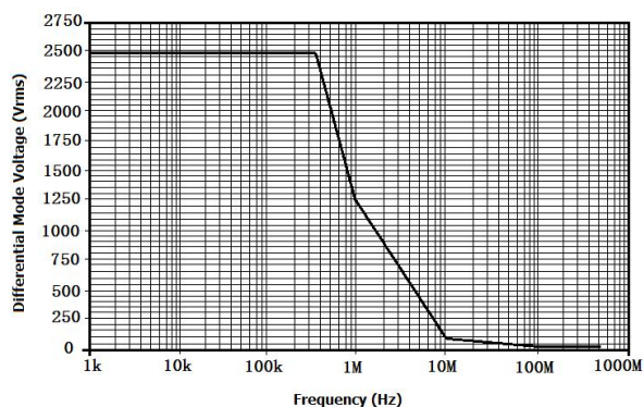
图 3 DPX6350B 最大差模电压 VS 频率
