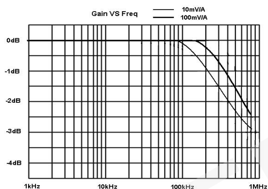
图 1 CPL8100A 典型增益频率关系曲线
