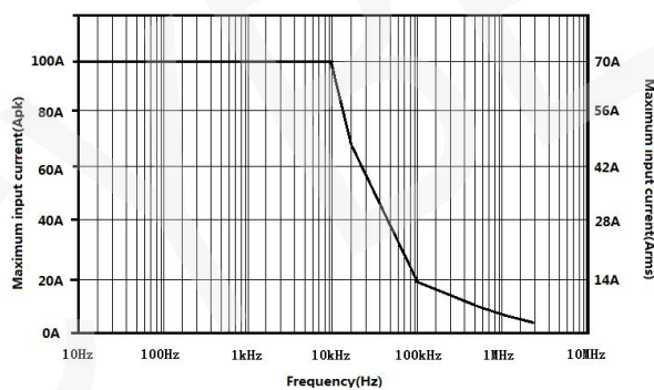
图 3 最大电流 VS 频率特性曲线
