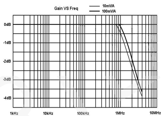
图 2 CPL8100B 典型增益频率关系曲线
