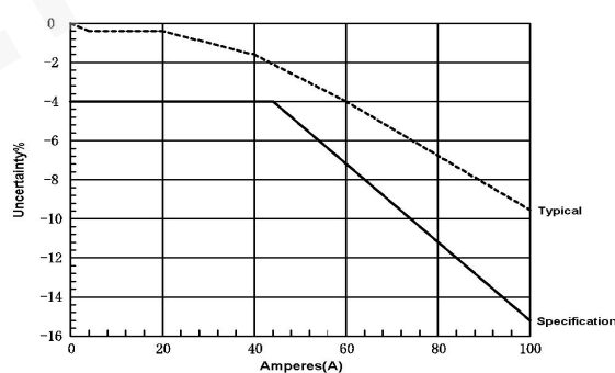
图 4 典型的 DC 线性度 (0.01V/A 档位)
