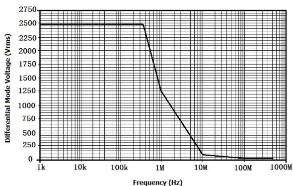
图 3 DP6350B 最大差模电压 VS 频率
