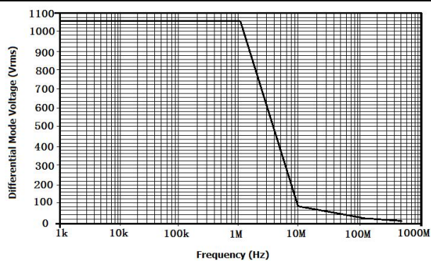
8 图 2 DP6150B 最大差模电压 VS 频率
