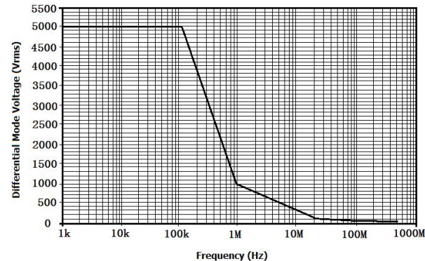
图 4 DP6700B 最大差模电压 VS 频率
