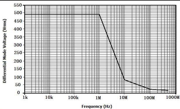
图 1 DP6070B 最大差模电压 VS 频率
